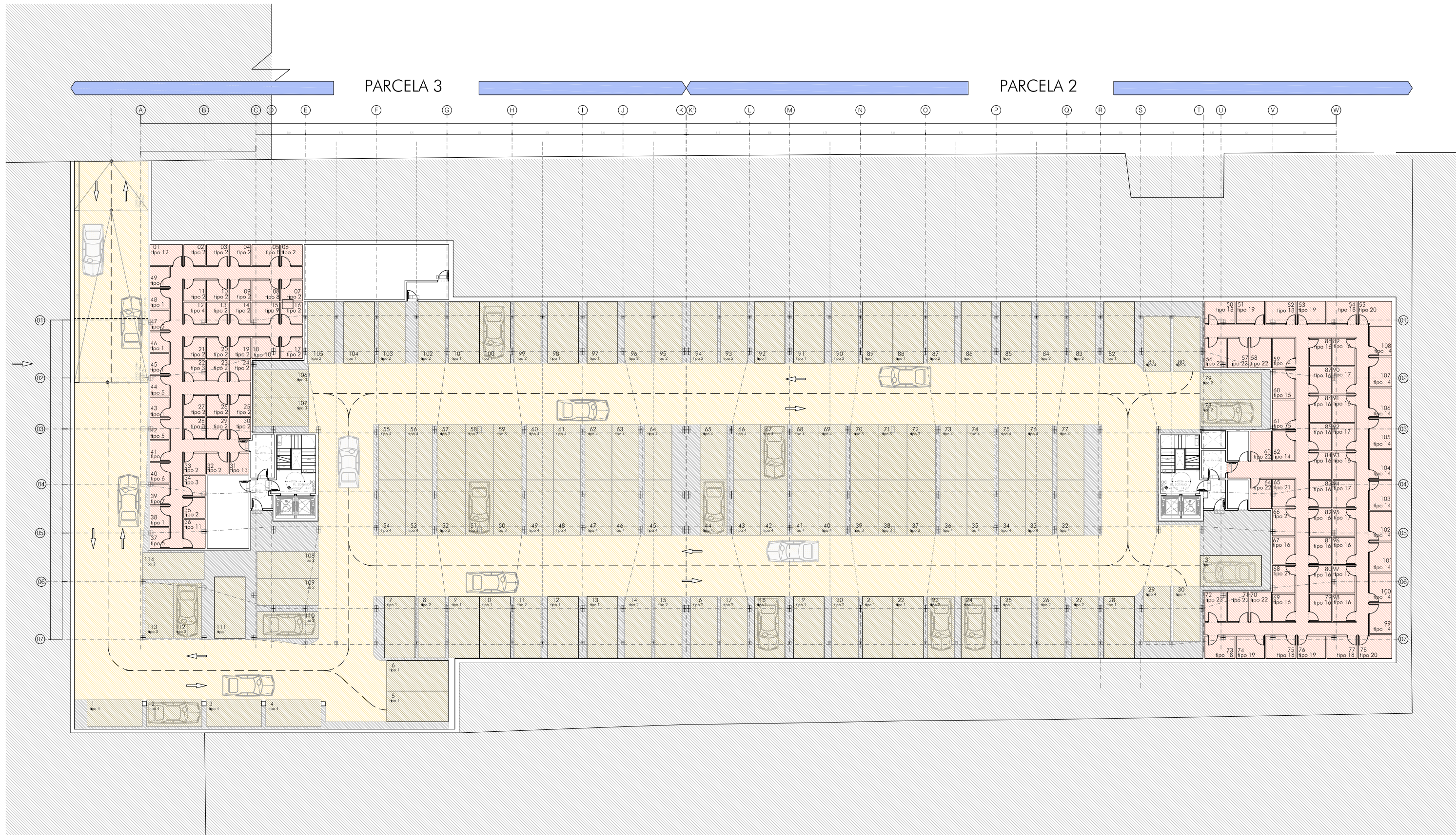
N PLANTA SOTANO 1/300
